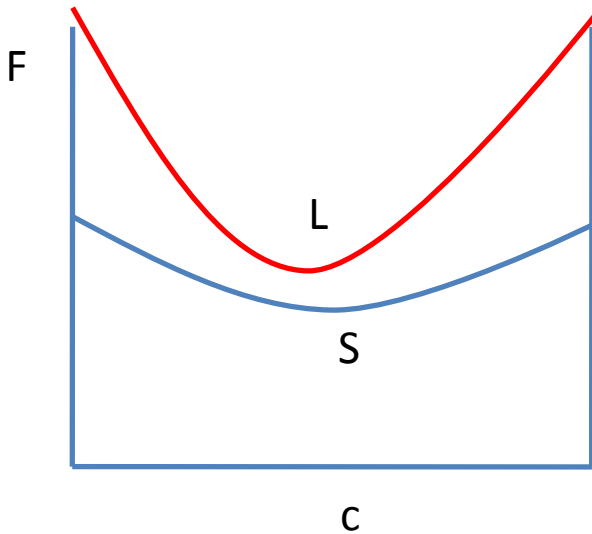
Free energy
