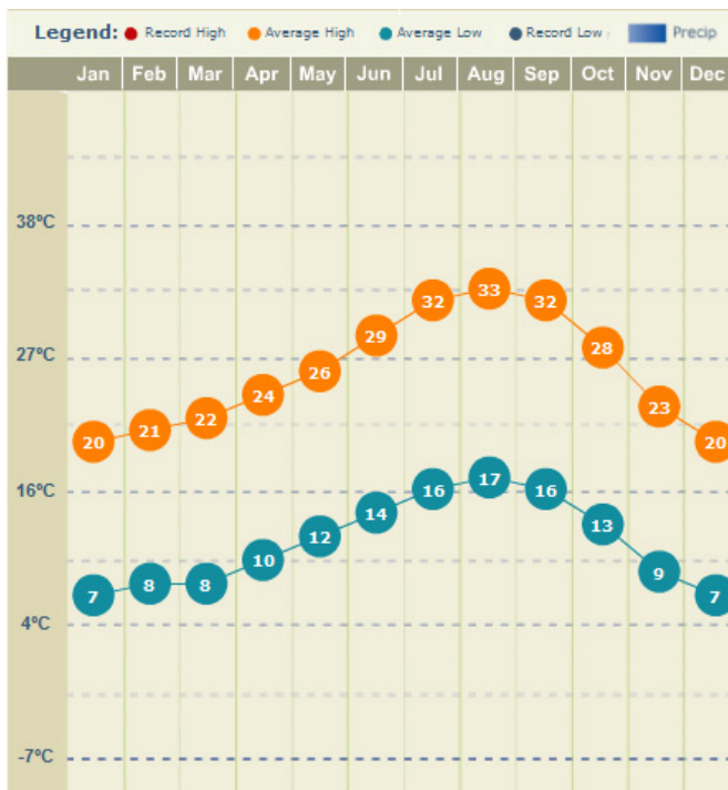
图为 Pasadena 的全年平均最高、最低气温曲线
